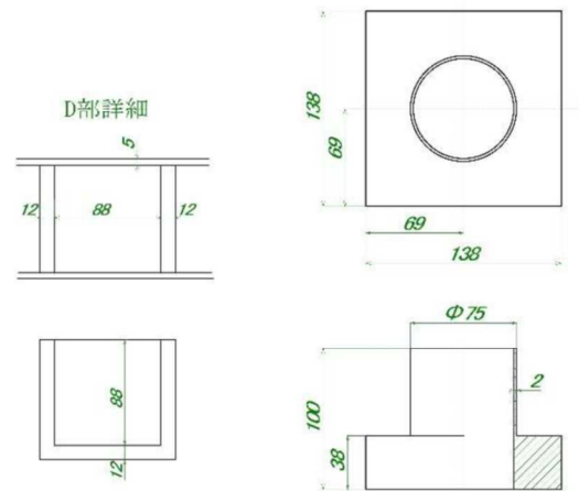
ゴールエリア2 詳細図
